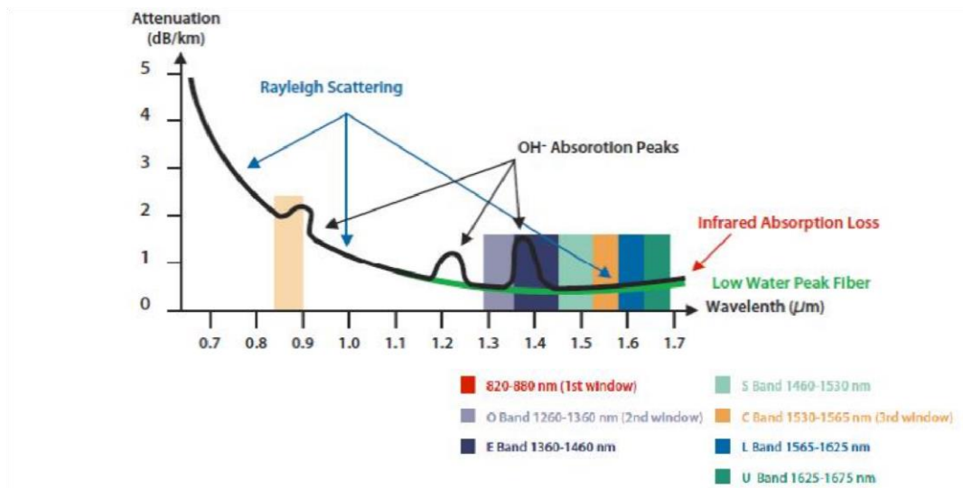
Figura 2.2 Ventanas y bandas de operación
