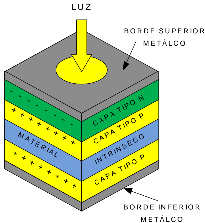
Figura 2.13 Estructura de un Fotodiodo APD
