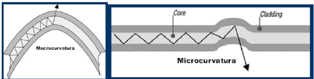
Figura 2.11 Atenuación debido a Macro y Micro curvaturas
