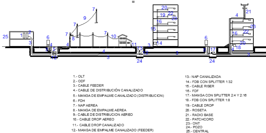
Figura 2.29 Elementos de la ODN
