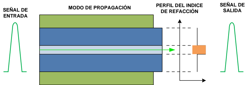
Figura 2.10 Fibra monomodo de índice escalonado
