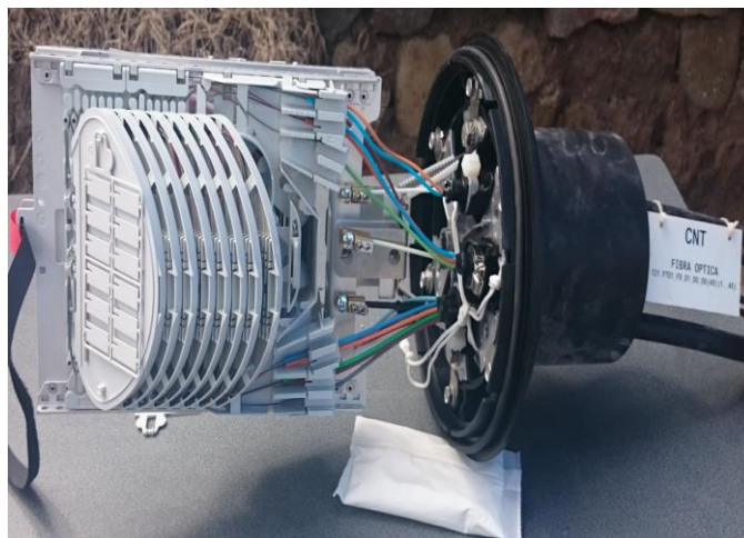
Figura 2.38 Manga de empalme de 96 Fibras Ópticas
