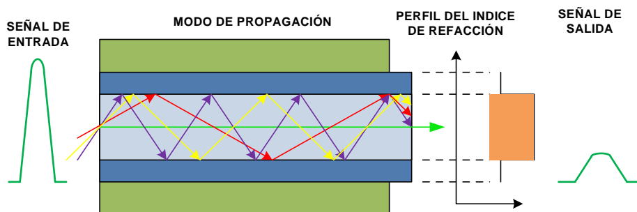
Figura 2.8 Fibra multimodo de índice escalonado
