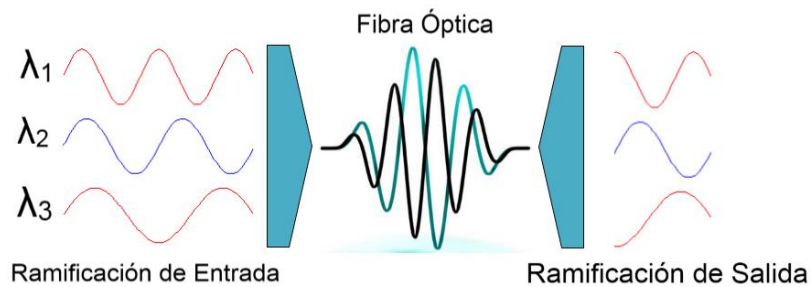
Figura 2.21 Multiplexación por División de Longitud de Onda
