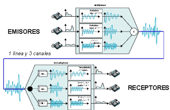
Figura 2.20 Multiplexación por División de Frecuencia
