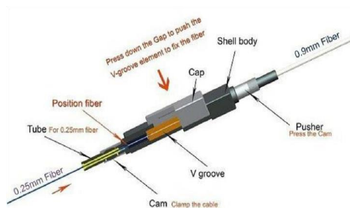
Figura 2.16 Estructura de un empalme mecánico
