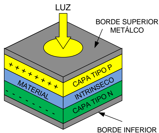
Figura 2.12 Estructura de un fotodiodo PIN
