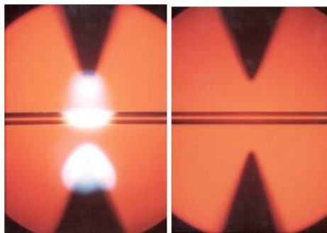
Figura 2.15 Método de empalme por fusión
