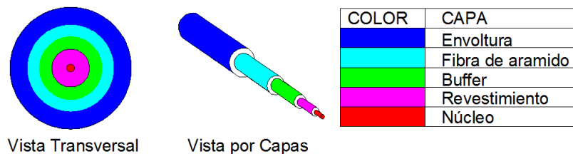
Figura 2.6 Estructura de la fibra óptica
