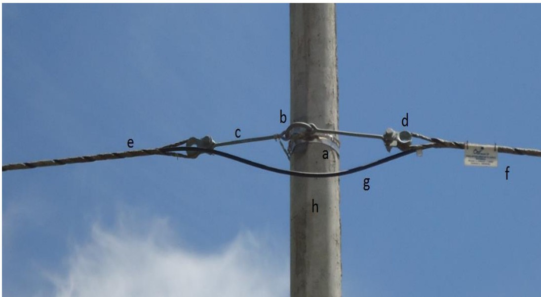
Figura 2.39 Herraje terminal
