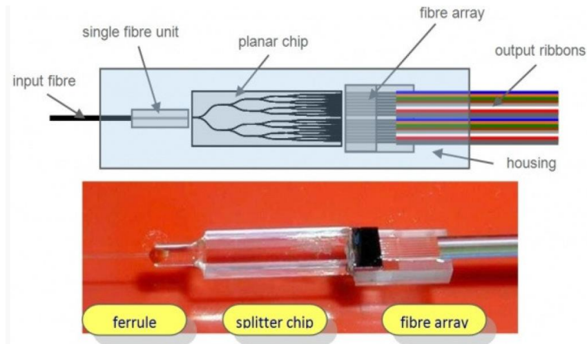
Figura 2.18 Fibra óptica Planar
