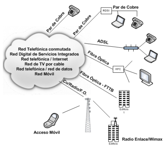
Figura 2.23 Diferentes tecnologías aplicadas en redes de acceso
