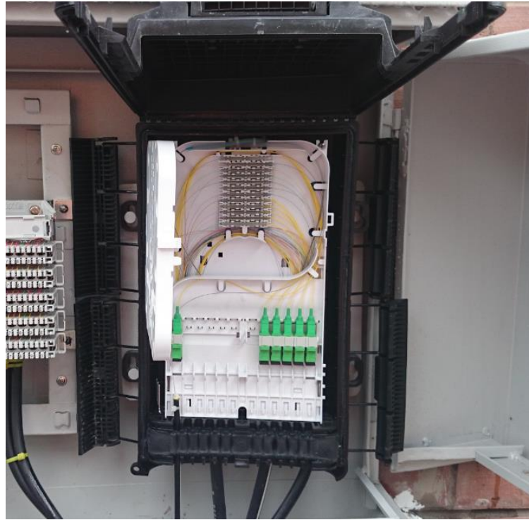
Figura 2.33 Caja de Distribución Óptica NAP
