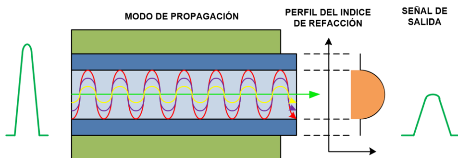
Figura 2.9 Fibra multimodo de índice gradual
