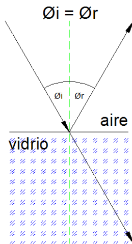
Figura 2.3 Ley de la reflexión de Snell
