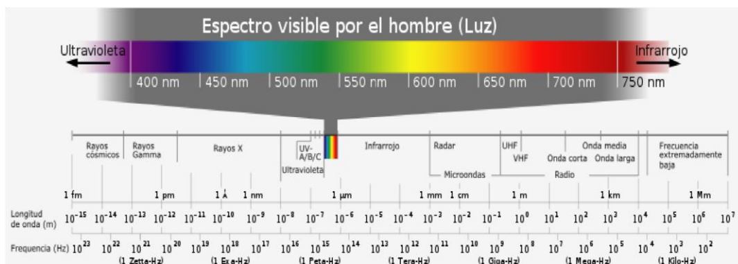
Figura 2.1 Espectro Electromagnético de la luz
