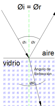
Figura 2.4 Ley de la Refracción
